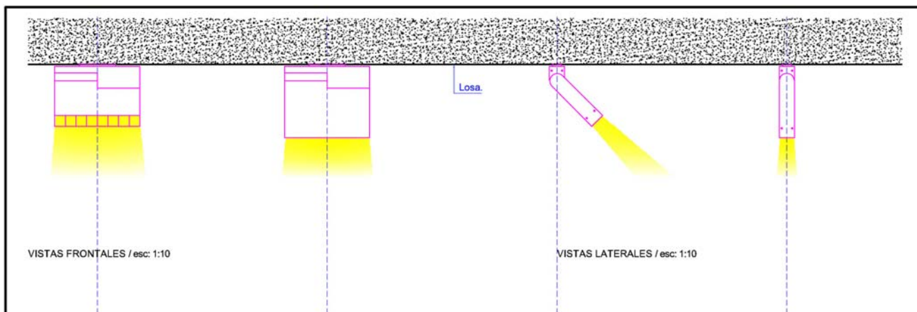
R13 ESQUEMA DE REFERENCIA / Luminaria tipo spot. / Sobrepuesta en losa o cielo. / Cripta.
