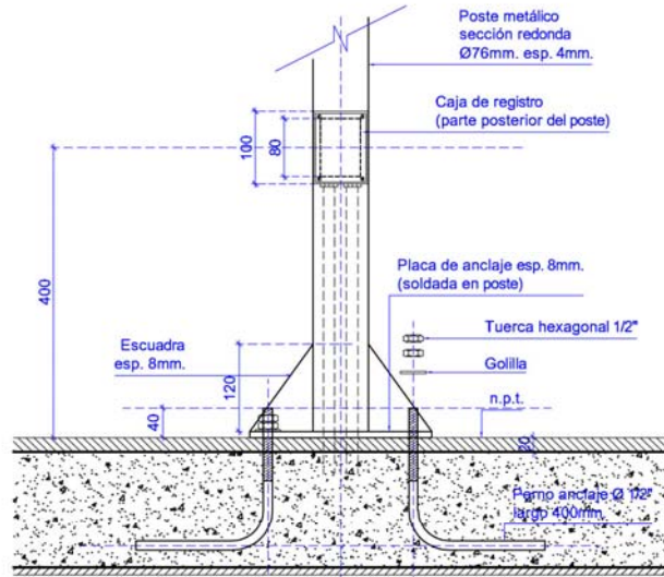
DETALLE ANCLAJE POSTE (EN LOSA) esc. 1:10
