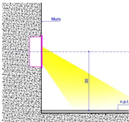
SECCION LATERAL / esc: 1:10
