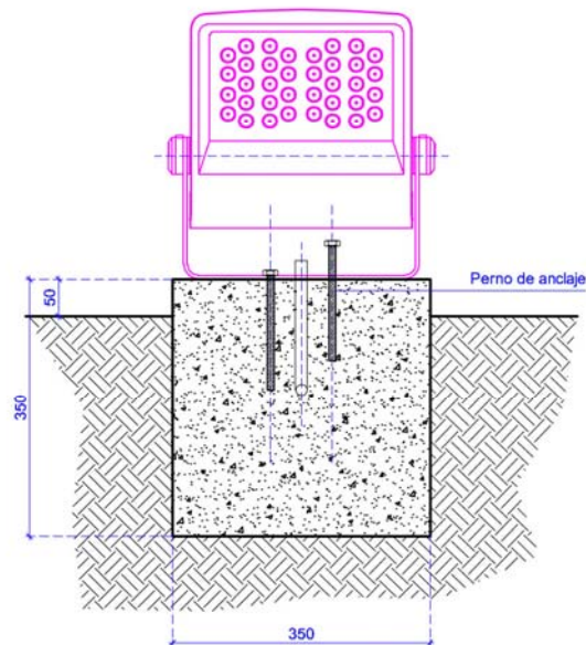
DETALLE DE ANCLAJE VISTA FRONTAL esc. 1:10
