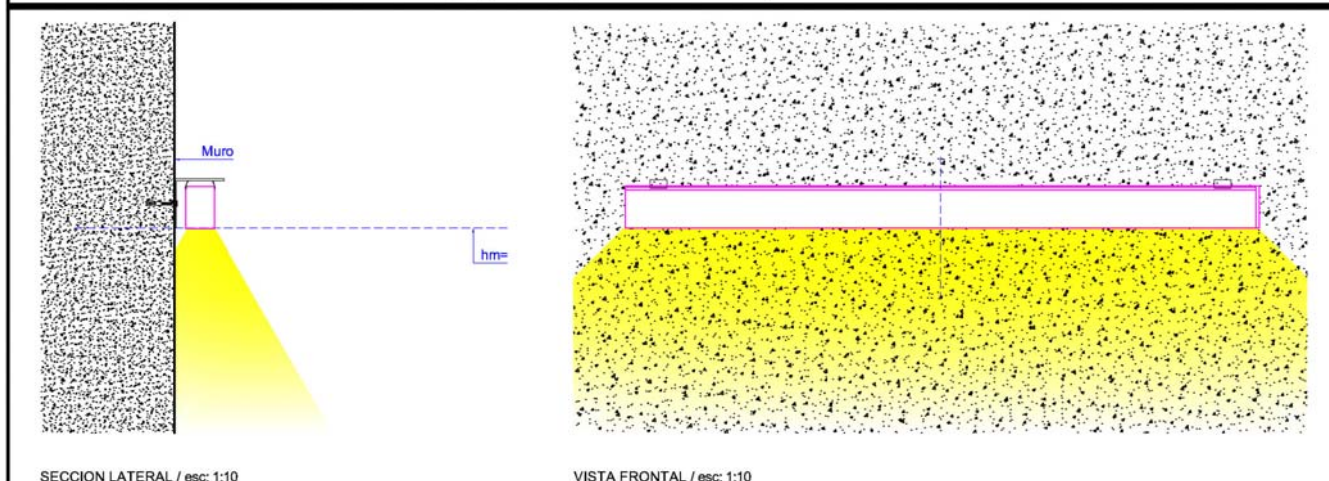
R14 ESQUEMA DE REFERENCIA / Luminaria lineal. / Adosada a muro. / Cripta.
