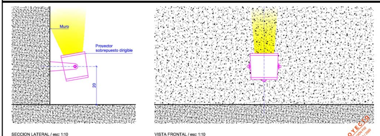
R15 ESQUEMA DE REFERENCIA / Luminaria spot tipo proyector. / Adosado a muro. / Fachadas.
