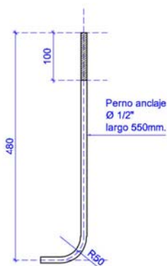
PERNO DE ANCLAJE esc. 1:10
