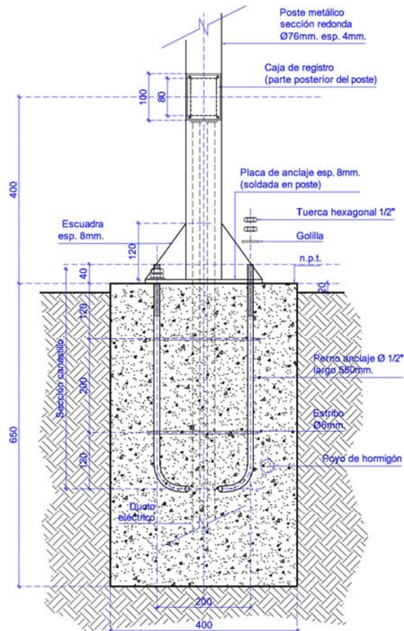
DETALLE ANCLAJE POSTE esc. 1:10
