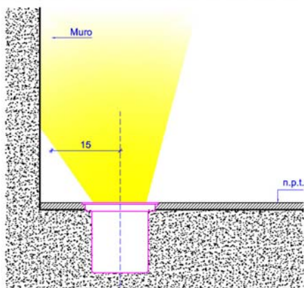
SECCION LATERAL / esc: 1:10
