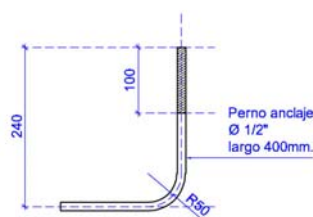
PERNO DE ANCLAJE esc. 1:10
