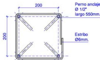
CANASTILLO DE ANCLAJE esc. 1:10
