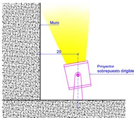
SECCION LATERAL / esc: 1:10
