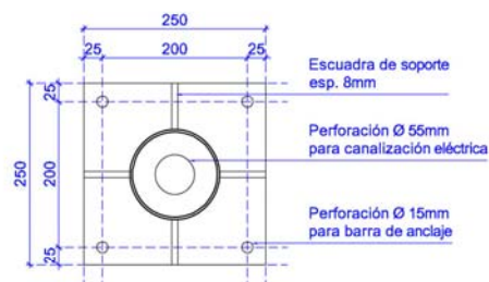
PLACA BASE DE ANCLAJE (Poste) esc. 1:10
