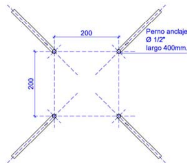
PERNOS DE ANCLAJE POSTE (EN LOSA) esc. 1:10
