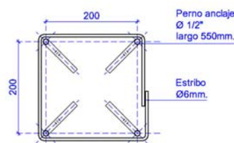
CANASTILLO DE ANCLAJE esc. 1:10
