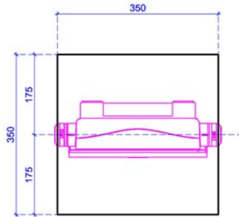
DETALLE DE ANCLAJE VISTA SUPERIOR esc. 1:10
